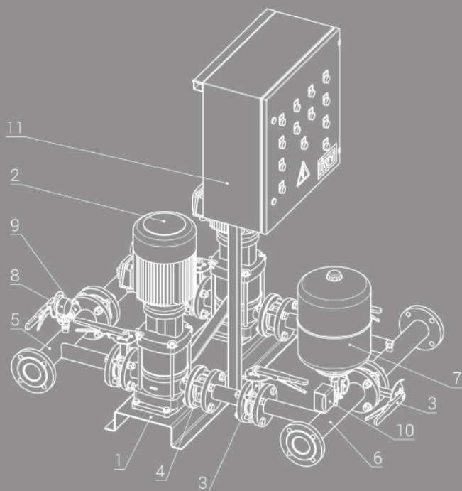
Насосна установка пожежогасіння Fire-Set DPV
